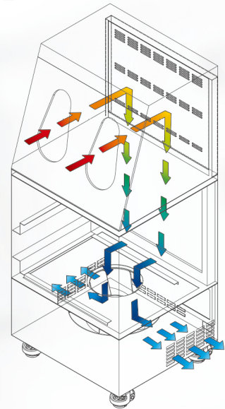
공기흐름도
